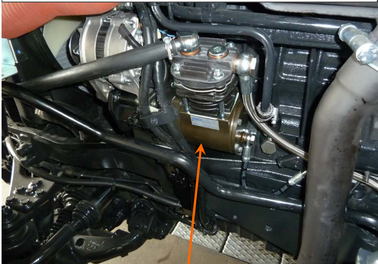
COMPRESSORE A TRASCINAMENTO A INGRANAGGI COMPRESSOR DRIVE GEAR
