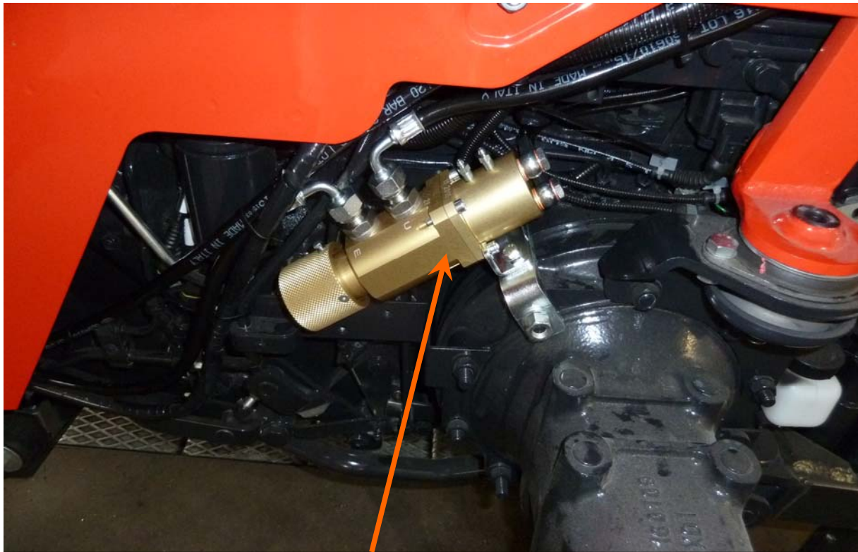
DISTRIBUTORE DI FRENATA CON REGOLAZIONE ANTICIPO/ RITARDO BRAKING DISTRIBUTOR WITH SETTING ADVANCE / DELAY
